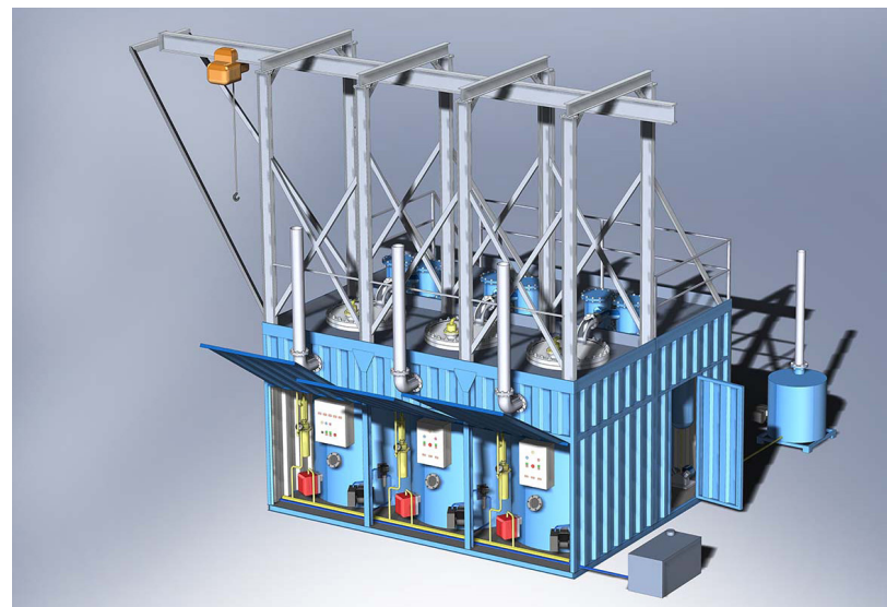
Модули пиролиза серий Фортан, МПК, МПВ, МПС
